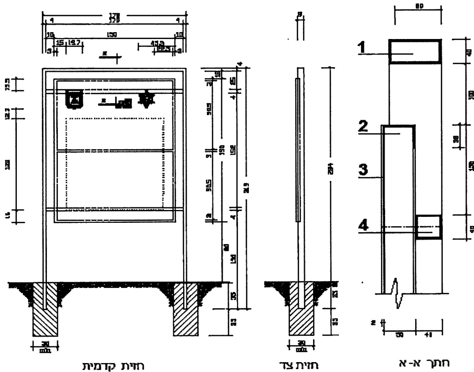
מידות - ע"פ תרשים ב-ס"מ
